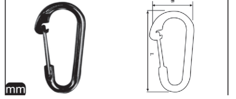
M 8007 Yaylı Karabina A4
