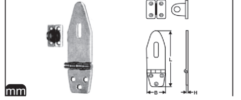
M 8052 A Kilit Köprüsü A2
