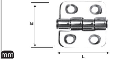
M 3838 Menteşe A2
