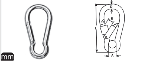
M 8249 Karabina A4
