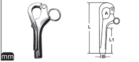
M 8157 Pelikan Kilit A4
