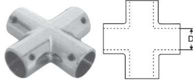
M 8387 Dörtlü Vardavela Bağlantısı A4
