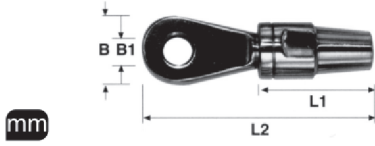
M 9213 Erkek Norsmen A2
