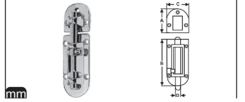
M 8333 Sürgü A2
