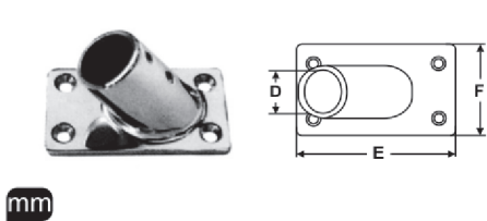
M 8204 Vardavela Ayağı Dikdörtgen Taban 60° A4
