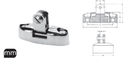
M 8573 Hareketli Tente Bağlantısı A4
