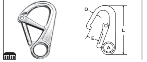
M 8338 Yaylı karabina A4
