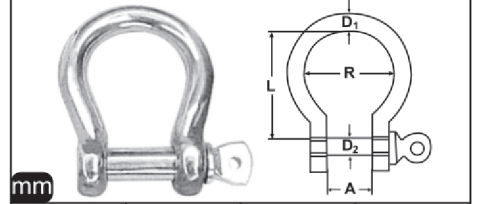
M 8260 Omega Kilit A4
