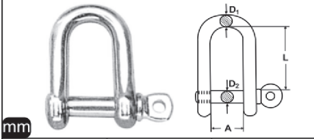
M 8258 Zincir Kilidi Kısa A4
