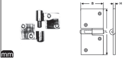
M 8239 Motor Kapak Menteşesi A4
