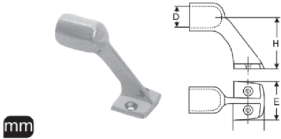
M 8213 Vardavela Tutamak Kapalı 60° A4
