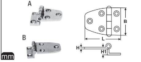
M 8237 Menteşe A4
