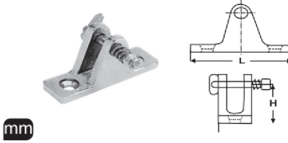
M 8328 Tente Bağlantısı Pimli A4
