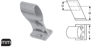
M 8207 Vardavela Ayağı Açık 60°
