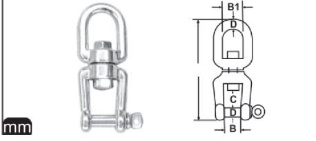
M 8255 Firdöndü Halka Kanca A4
