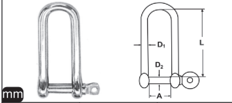
M 8259 Zincir Kilidi Uzun A4
