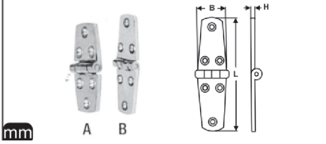
M 8280 Menteşe A4
