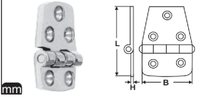
M 8234 Menteşe A4
