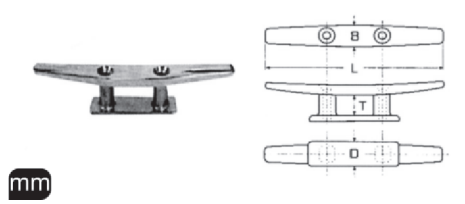
M 8298 Koç Boynuzu Üstten Vidalı A4
