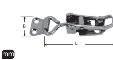
M 8427 Ayarlı Gergi Kilidi
