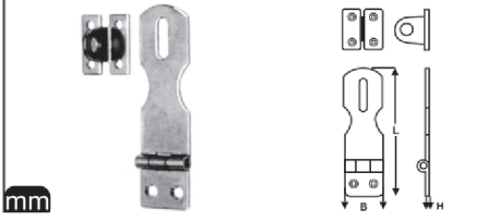
M 8052 Kilit Köprüsü A2
