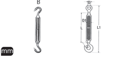
M 8246 B Liftin Kanca Kanca A4
