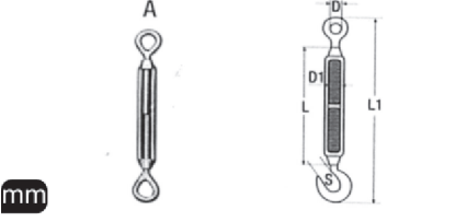
M 8246 A Liftin Halka Halka A4
