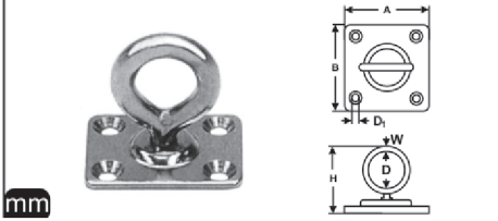
M 8396 Dönerli Mapa A2
