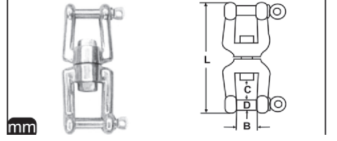
M 8256 Firdöndü Kanca - Kanca A4
