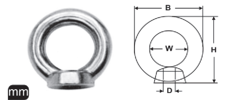
D 582 Halkalı Somun
