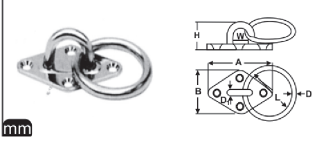
M 8265 Halkalı Mapa A2
