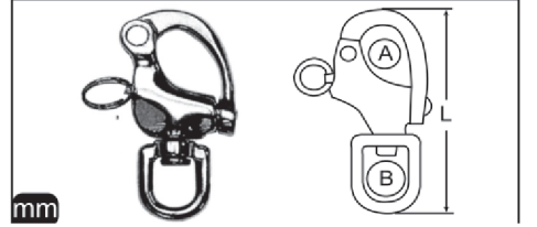
M 8252 Mandar Kilidi A4
