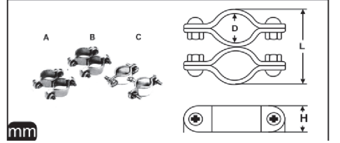
M 8461 Çiftli Kelepçe A4
