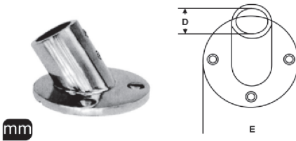
M 8202 Vardevela Ayağı 60° A4
