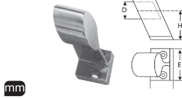
M 8208 Vardavela Ayağı Kapalı 60°
