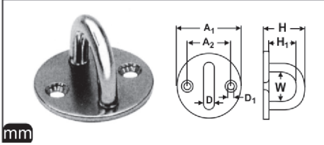
M 8253 Yuvarlak Mapa A2
