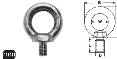
D 580 Halkalı Civata
