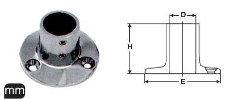
M 8201 Vardavela Ayağı 90° A4
