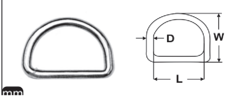
M 8376 D Halka A4
