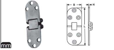
M 8018 Masa Menteşesi A4
