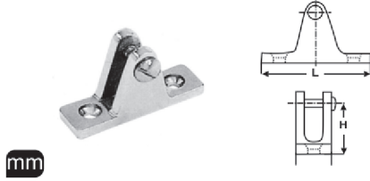
M 8273 Tente Bağlantısı Vidalı A4
