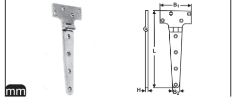
M 8281 T Menteşe A4
