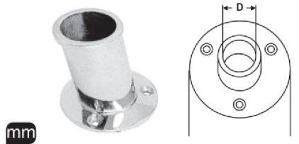
M 8283 Bayrak Direği Tutucusu 84° A4
