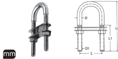
M 8230 U Mapa Kademeli
