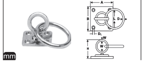
M 8397 Dönerli Halkalı Mapa A2
