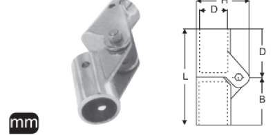
M 8572 Boru Mafsalı
