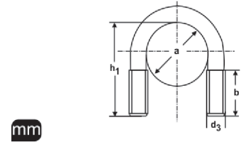
DIN 3570 U Bolt
