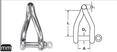
M 8288 Burgu Kilit A4
