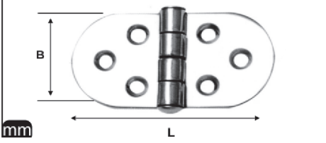
M 3871 Menteşe A2
