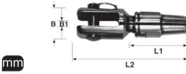
M 9214 Dişi Norsmen A2
