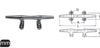
M 8217 Koç Boynuzu Yuvarlak A4
