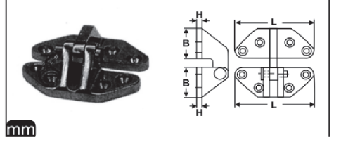
M 8238 Kapak Menteşesi A4
