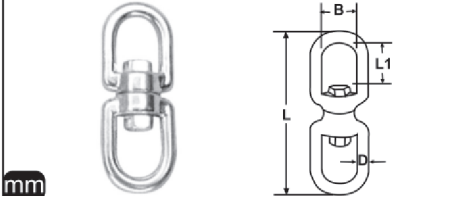
M 8254 Firdöndü Halka - Halka A4
