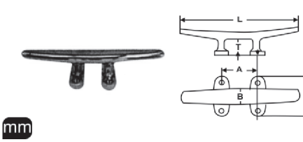
M 8218 Koç Boynuzu Yassı A4
