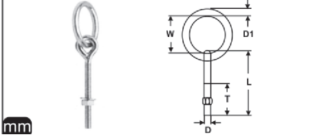
M 8228 Halkalı Vidalı Mapa A4
