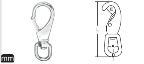
M 8257 Firdöndülü Karabina A4
