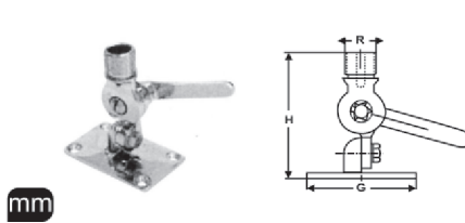
M 8279 Anten Tutucu
