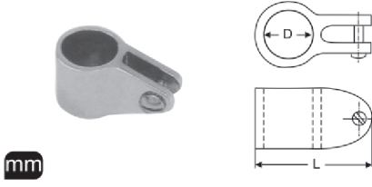
M 8271 Tente Boru Geçişi A4
