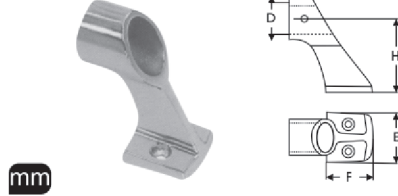
M 8276 Vardavela Tutamak Açık 60° A4
