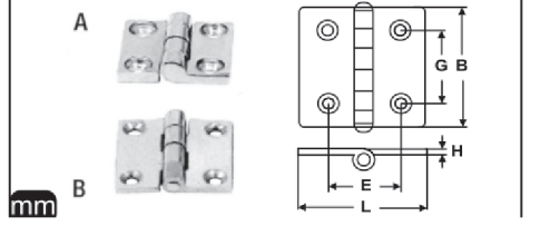
M 8233 Menteşe A4
