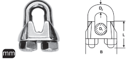
M 8248 Klemens A4
