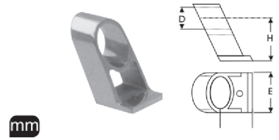
M 8209 Vardavela Tutamak Açık 60°
