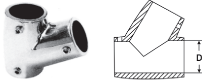
M 8206 Vardavela T 60°
