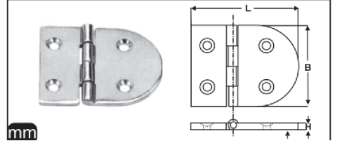
M 8429 Menteşe A4
